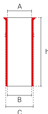
CAZOLETAS HERMETICA H 240 BOCAIS HERMETIC H 240 Consulte la página - Ver pág.22
