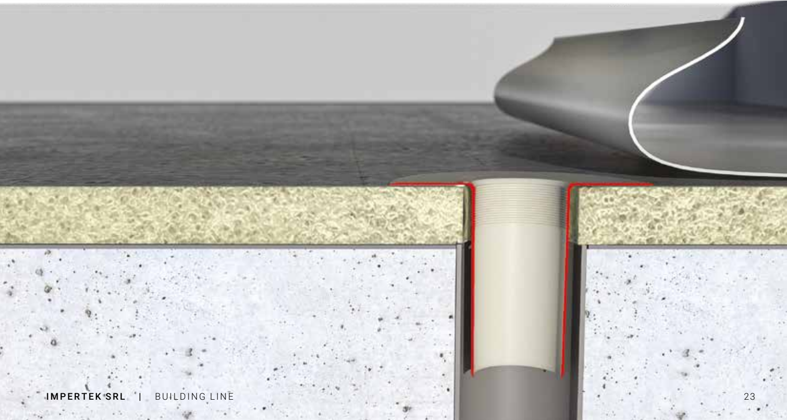
EJEMPLO DE COLOCACIÓN DE CAZOLETAS ERMETIC DE PVC CON LÁMINAS SINTÉTICAS EXEMPLOS DE COLOCAÇÃO BOCAIS ERMETIC EM PVC COM TELAS SINTÉTICAS
