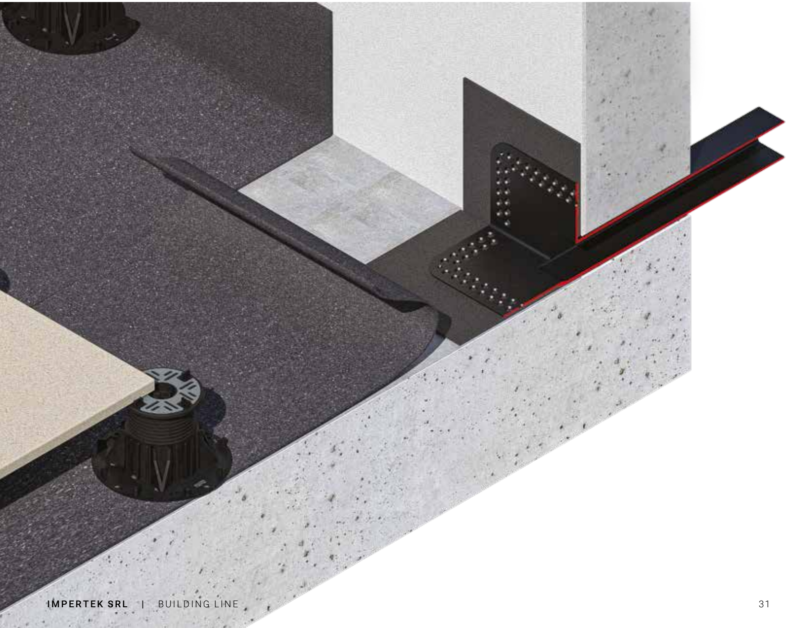
EJEMPLO DE COLOCACIÓN DE SALIDAS DE TPE CON MEMBRANAS BITUMINOSAS EXEMPLOS DE COLOCAÇÃO BOCAIS ANGULARES EM TPE COM MEMBRANAS BITUMINOSAS
